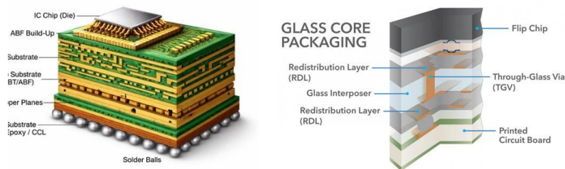
圖二、玻璃基板 GCS 結構
